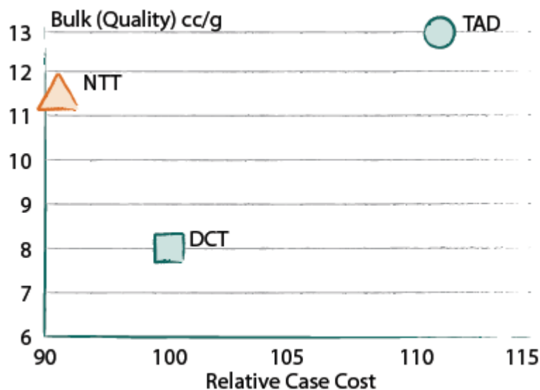
Figur 3 visar sammenhanget mellom bulk (uttryckt for papprets vikt og tjocklek) og relativ utgift. Jämförelse mellan 3 teknologier: Den nya NTT-teknologin, DCT avancerad yankeemaskin och konventionell TAD vid produktion av toalettpapper 20-22 g (inklusive energi, kemikalier, massa och vid detta tillfälle en besparing på 15 % fibrer för NTT och DCT ( www.metsopaper.com )).
